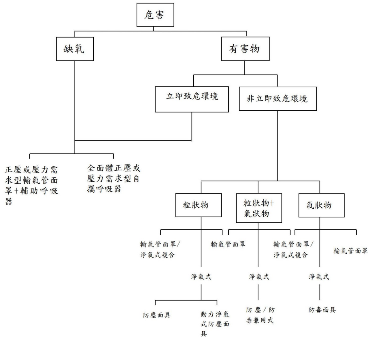
附表二:呼吸防護具選用步驟
